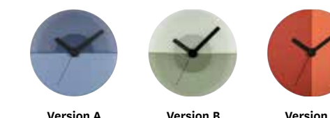
Horloge TOLIX Time NEW Design : Kilian Schindler H.85 x Ø450 mm / 4,50 kg Coloris du verre : Naturel ou Argent Pile / Battery : AA - 1,5 V - LR6 (non fournie / not included) Disponible en version couleurs personnalisables. Available in customizable colors. TOLIX maison
